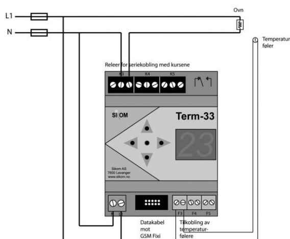
Exempel på anslutning.
